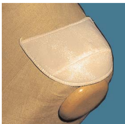
Art. W 640 Schulterpolster, Soft, R Überzug: IV Größe: 120x80x5mm col.: weiß, schwarz VE: 10 Paar
